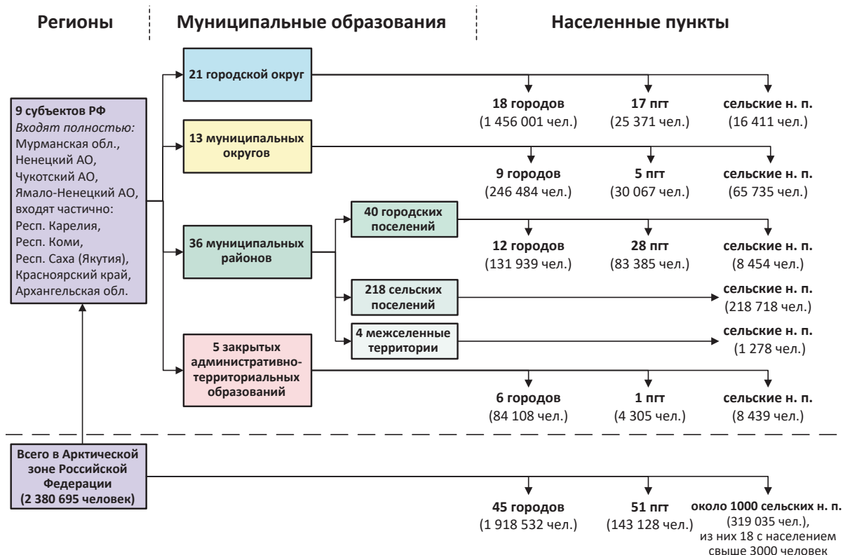
Рис. 1. Административное деление российской Арктики и распределение населения по типам населенных пунктов (перепись населения 2021 г.)
